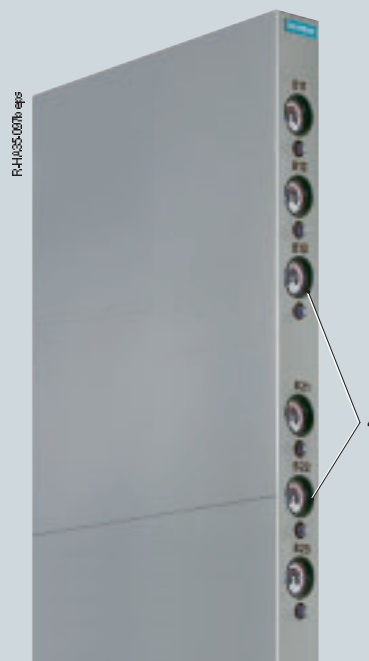
Манометры (4) на фазы сборных шин (расположены в боковой конечной стенке КРУЭ)
