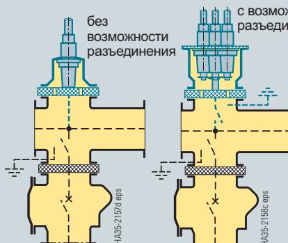
Подключение для сборных шин
