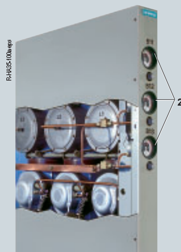
Манометры (2) на фазы сборных шин (расположены в боковой конечной стенке КРУЭ (боковая стенка открыта))
